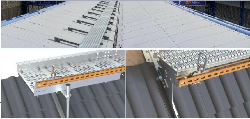
C-Schiene 500
