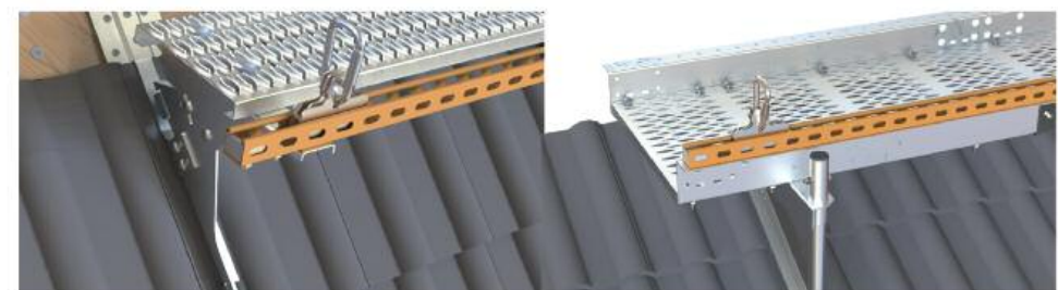
C-Schiene 250
